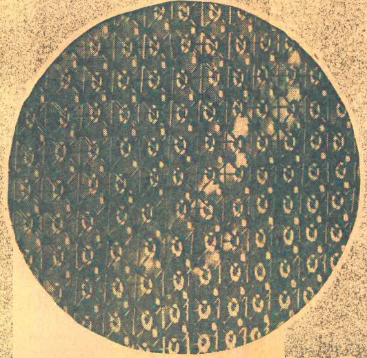
Foto ampliada de la matriz de una memoria. Cada uno de estos anillos o tirrosos puede estar magnetizado en una u otra dirección con lo que se consigue la más variada combinación de datos.
